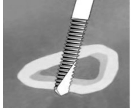
Рис. 22-6. 5-мм стержень після проходження крізь два шари щільної речовини кістки.
