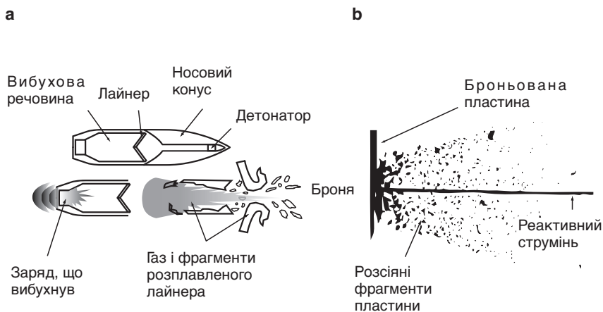
Рис. 1-8. (а) Механізми, через які бойова головка кумулятивного заряду викликає руйнування. (b) Діаграма, яку було зроблено з фотографії реальної детонації бойової головки кумулятивного заряду при зіткненні з броньованою пластинною.
