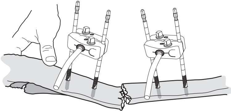
Рис. 22-12. Встановлення другого багатостержневого тримача з двома стержнями. Під'єднайте 30-градусні колінця до двох багатостержневих тримачів. Спрямуйте колінця у напрямку, в якому зовнішні опори будуть міститися якомога далі від відкритих ран і не перешкоджатимуть їх догляду.
